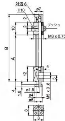
バッファ付外形寸法図
