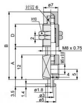
バッファ付外形寸法図
