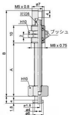
バッファ付外形寸法図
