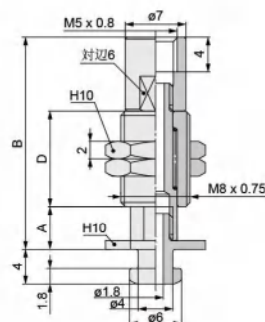
バッファ付外形寸法図
