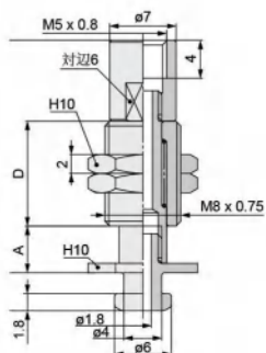
バッファ付外形寸法図
