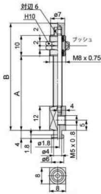
バッファ付外形寸法図
