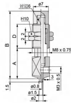
バッファ付外形寸法図
