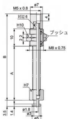
バッファ付外形寸法図
