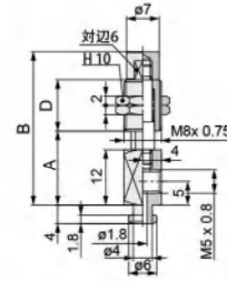
バッファ付外形寸法図
