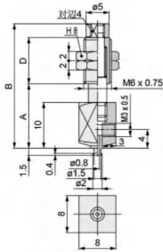
バッファ付外形寸法図
