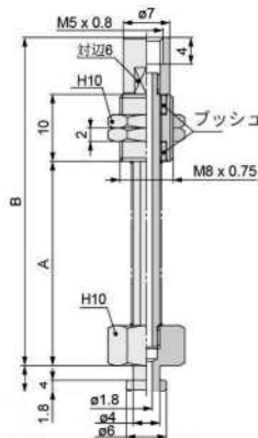
バッファ付外形寸法図
