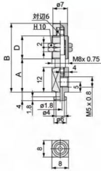
バッファ付外形寸法図
