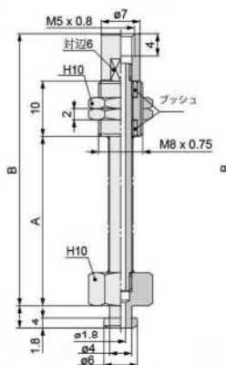
バッファ付外形寸法図
